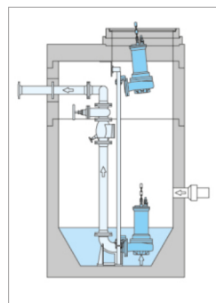
永久湿井安装
