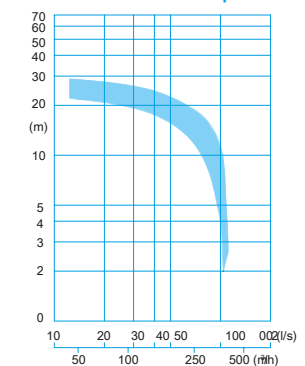
CK 33... -4 pole
