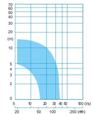
CV(X) 23... -4 pole
