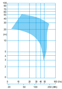
CMX 23... -2 pole
